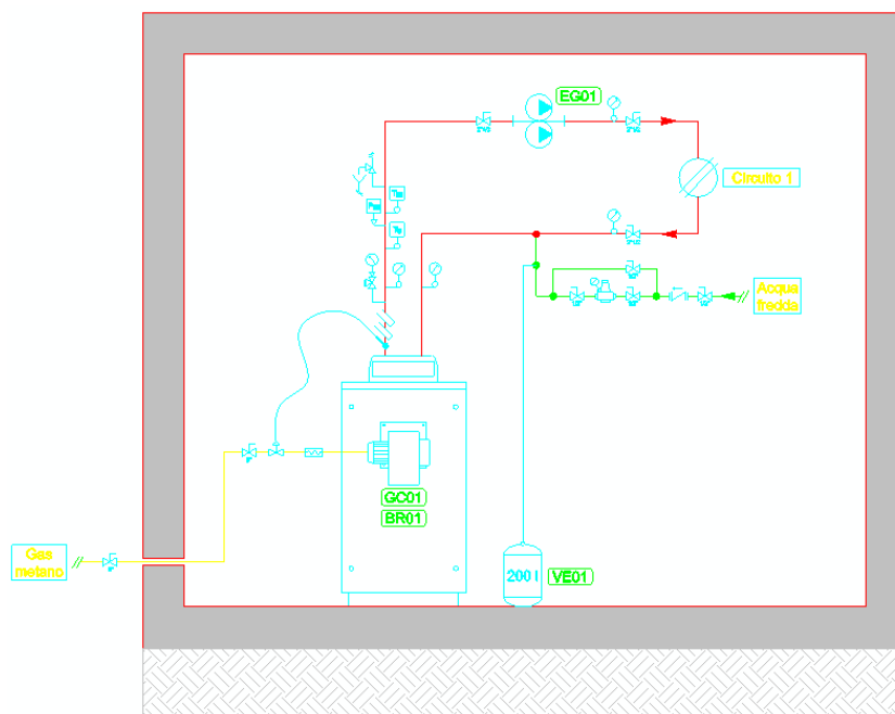
Figura 4.7 - Particolare dello schema di impianto
