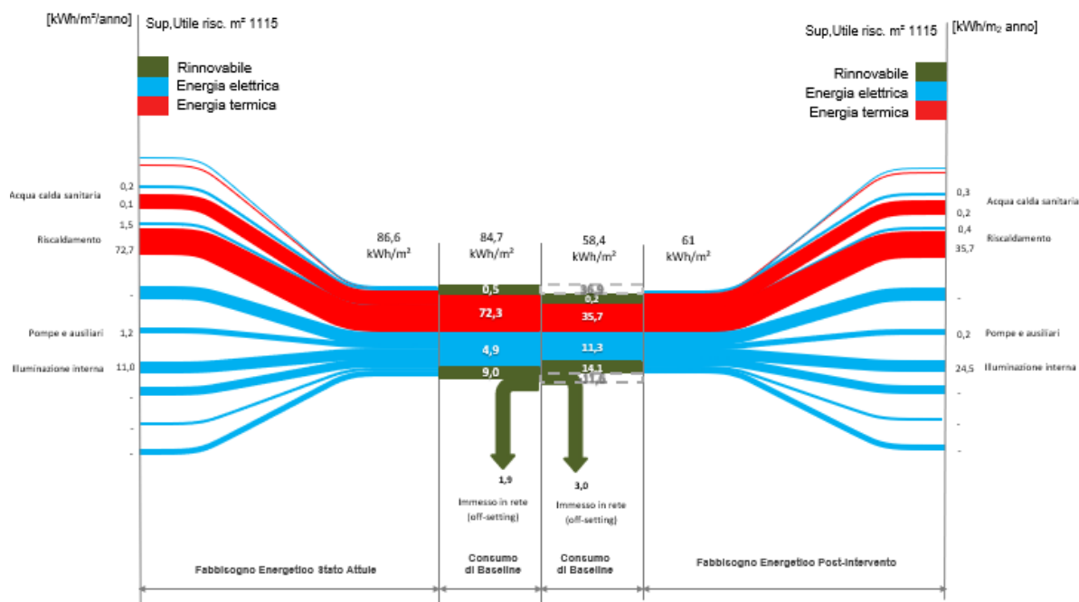
Figura 9.20 – SCN1: Bilancio energetico complessivo dell’edificio post intervento
