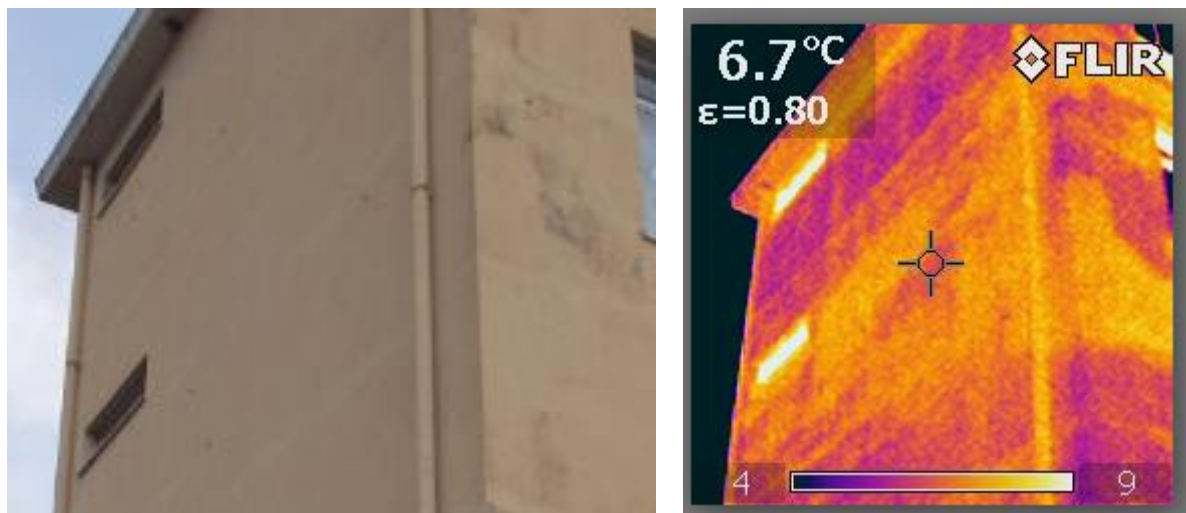
Figura 4.3 – Rilievo termografico della parete
