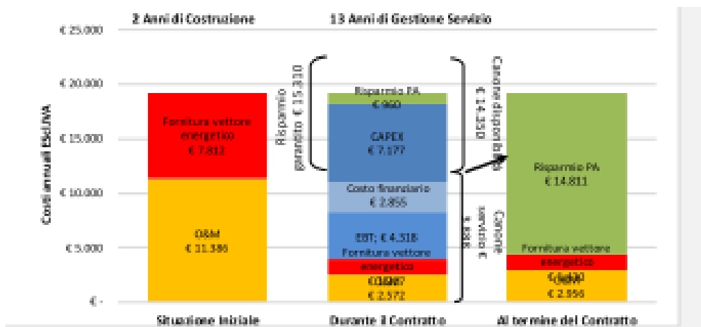
Figura 9.24 – Scenario 1: Schema di Energy Performance Contract
